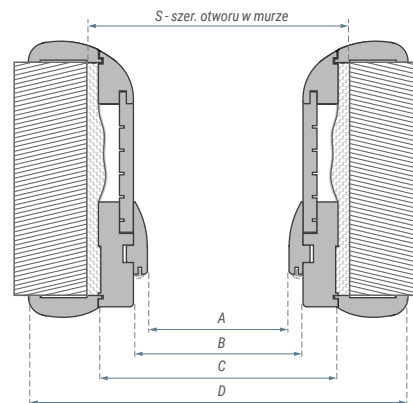
Wymiary ościeznicy New Arcus [mm]:
