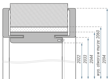
▼ Wymiary ościeżnicy do drzwi Natura HK PN22.
