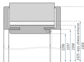
▼ Wymiary ościeżnicy do drzwi Natura HK PN23.
