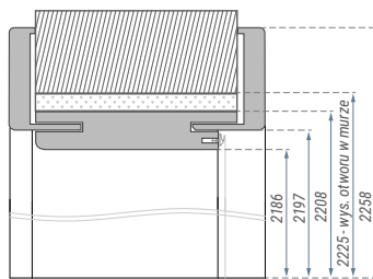
▼ Wymiary ościeżnicy do drzwi Natura HK PN22.
