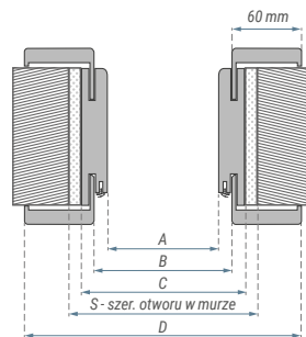
▼ Wymiary ościeżnicy do drzwi Natura HK PN23.
