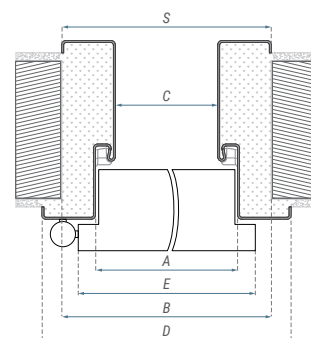
Wymiary ościeżnicy drewnianej PPOŻ [mm]
